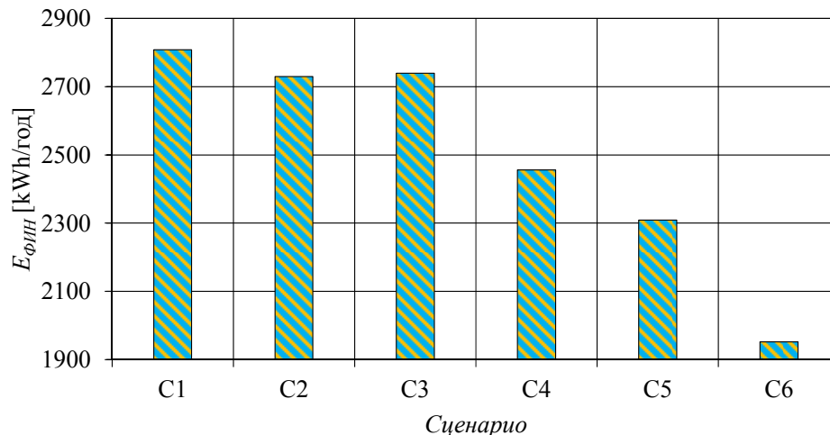
Сл. 5 – Потрошња финалне (електричне) енергије током анализираних периода у различитим типовима подземних зграда (C2-C6) у односу на надземну зграду (C1) / Fig. 5 – Final (electrical) energy consumption during the analyzed period in different underground building types (S2-S6) in relation to the above-ground building (S1)
