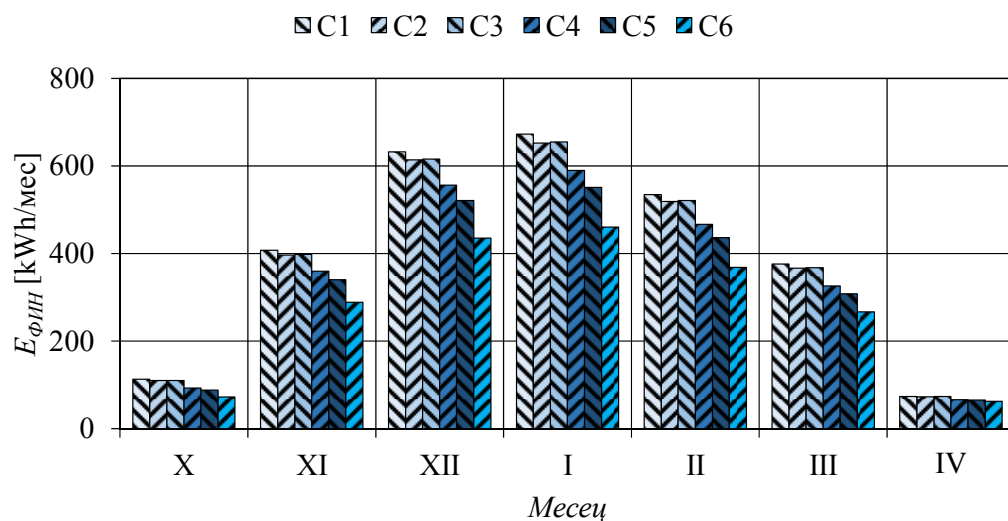
Сл. 6 – Месечна потрошња финалне (електричне) енергије током анализираних месеци у различитим типовима подземних зграда (С2-С6) у односу на надземну зграду (С1) / Fig. 6 – Monthly final (electrical) energy consumption during the analyzed period in different underground building types (S2-S6) in relation to the above-ground building (S1)
