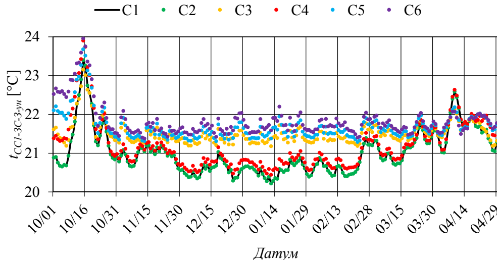
Сл. 9 – Просечна дневна температура западног спољашњег зида са унутрашње стране у спаваћој соби 1 током анализираниг периода у зависности од испитаног сценарија (C1-C6) / Fig. 9 – Average daily temperature of the west exterior wall on the inside of bedroom 1 during the analyzed period, depending on the scenario (S1-S6)
