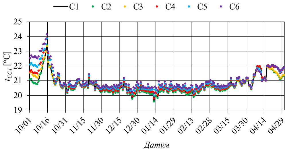
Сл. 7 – Просечна дневна температура у спаваћој соби 1 током анализираниг периода у зависности од испитаног сценарија (C1-C6) / Fig. 7 – Average daily temperature in bedroom 1 during the analyzed period depending on the scenario (S1-S6)
