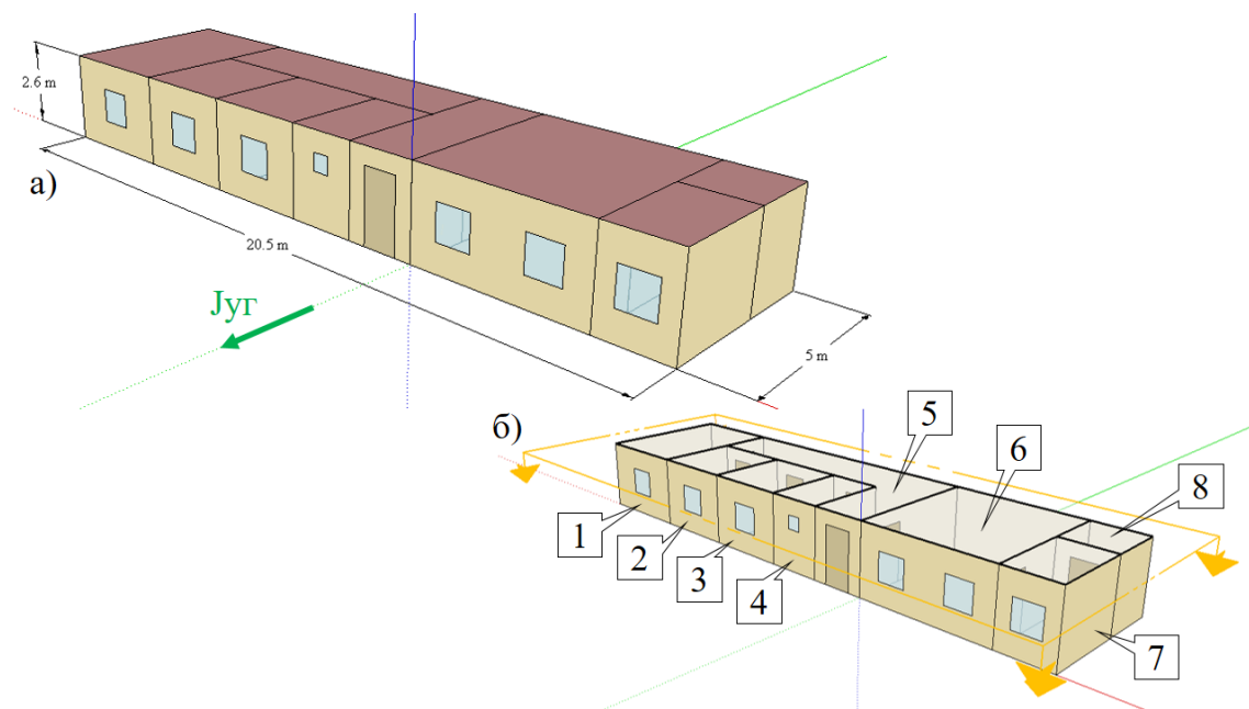
Сл. 1 – Предмет нумеричког истраживања: а) Изометријски приказ; б) Распоред просторија; (1) Спаваћа соба 1; (2) Спаваћа соба 2; (3) спаваћа соба 3; (4) Купатило; (5) Ходник; (6) Дневна соба; (7) Кухиња; (8) Остава / Fig. 1 – The subject of numerical investigation: a) Isometric view; b) Rooms layout; (1) Bedroom 1; (2) Bedroom 2; (3) Bedroom 3; (4) Bathroom; (5) Hall; (6) Living room; (7) Kitchen; (8) Pantry
