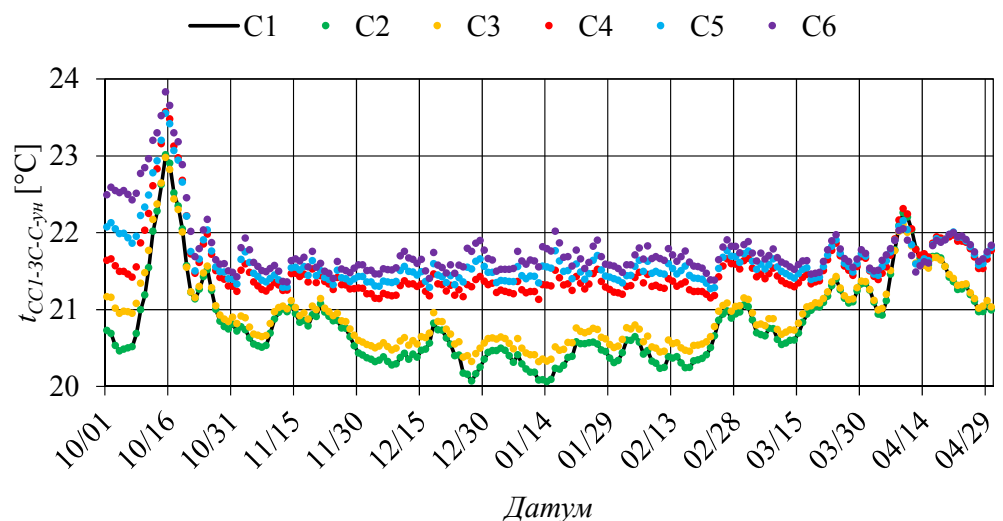
Сл. 8 – Просечна дневна температура северног спољашњег зида са унутрашње стране у спаваћој соби 1 током анализираниг периода у зависности од испитаног сценарија (C1-C6) / Fig. 8 – Average daily temperature of the north exterior wall on the inside of bedroom 1 during the analyzed period depending on the scenario (S1-S6)
