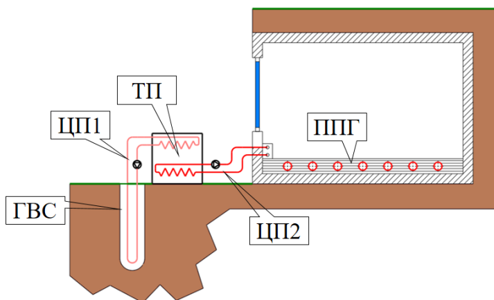
Сл. 2 – Шема рада топлотне пумпе земља-вода: ТП – Топлотна пумпа земља-вода; ГВС – Геотермална вертикална сонда; ЦП1 – Циркулациона пумпа 1; ЦП2 – Циркулациона пумпа 2; ППГ – Подни панелни грејач / Fig. 2 – Operation scheme of the ground source heat pump: GSHP – Ground source heat pump; GVP – Geothermal vertical probe; CP1 – Circulation pump 1; CP2 – Circulation pump 2; FPH – Floor panel heater
