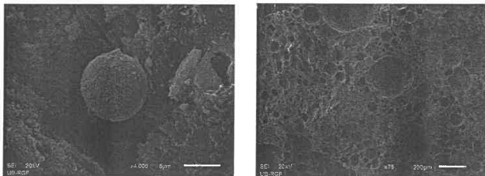
Slika 5. Mikrostruktura betona
