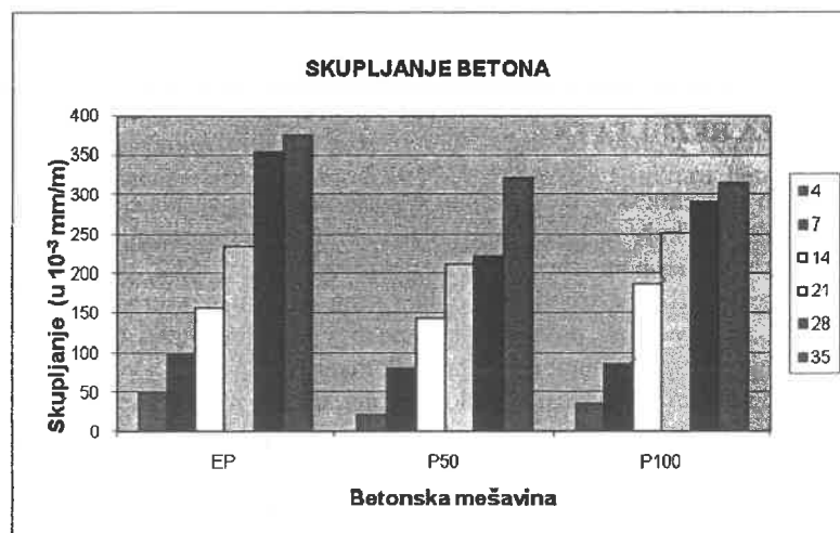
Slika 4. Skupljanje betona
